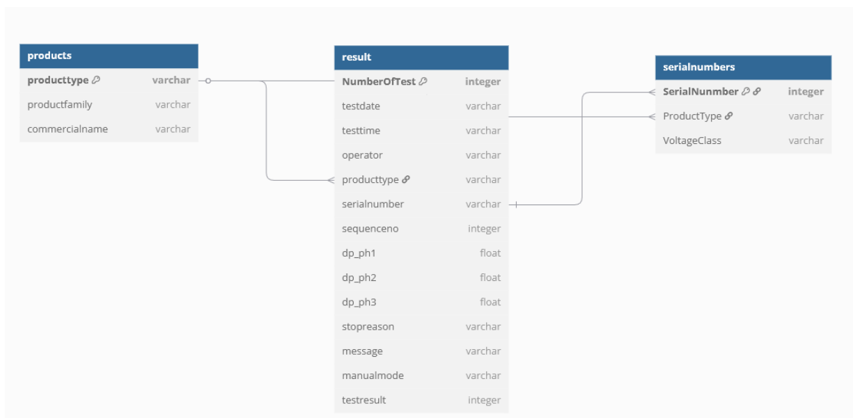
Diagramme de classes
